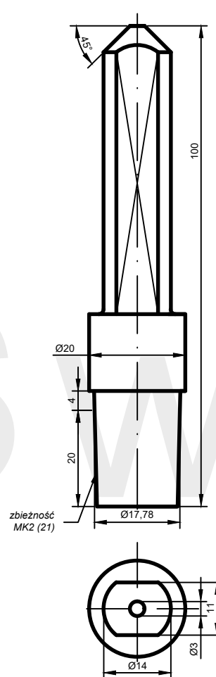
AW: B1(3)-20(14x11).100-21*
