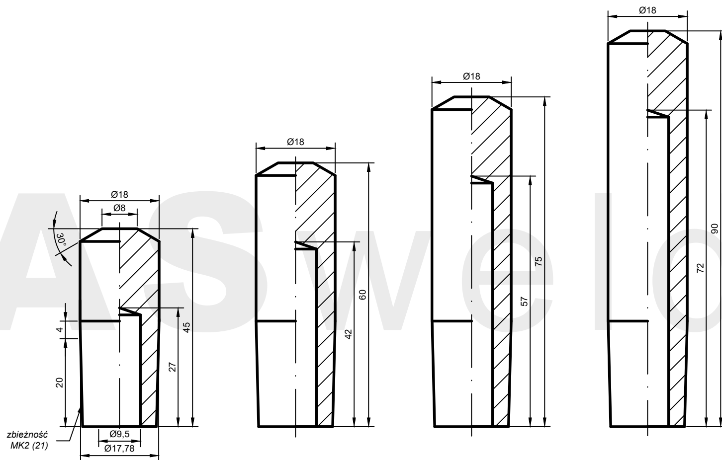
AW: B(8)-18.45-21*
