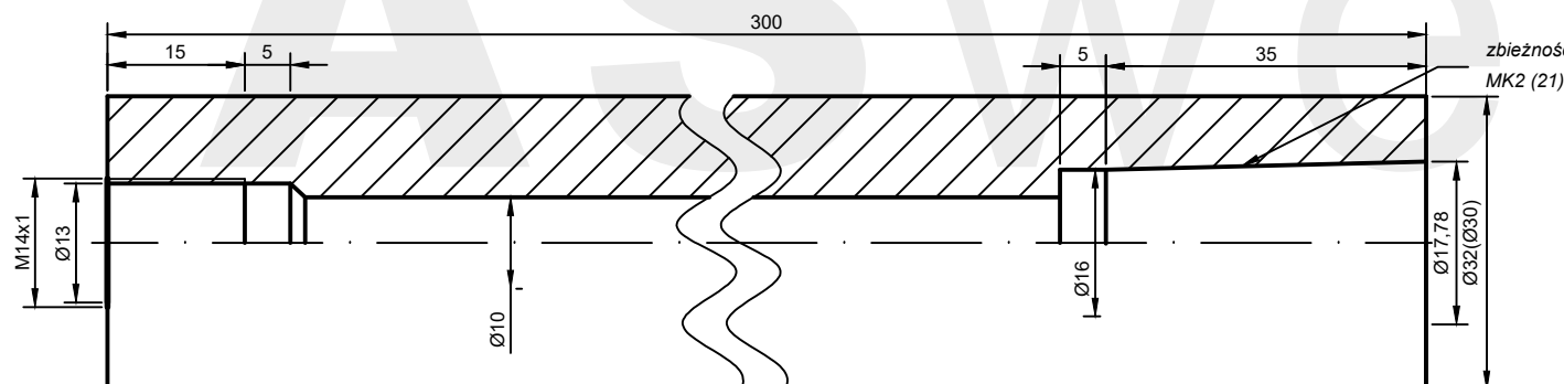
AW: S_21-32(Ø30).300
