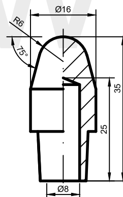
AW: E3(6)-16.35-40
