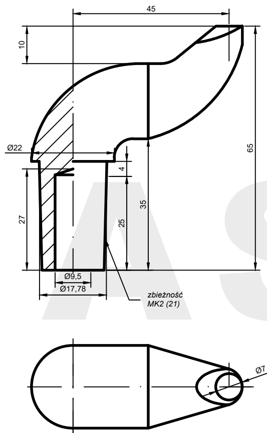
AW: F07(7)-22.65.45-21
