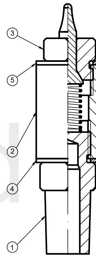
Elektroda z pinem do automatycznego podawania nakrętek
