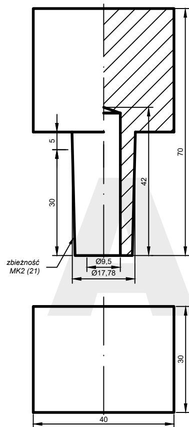
AW: C-30x40.70-21*
