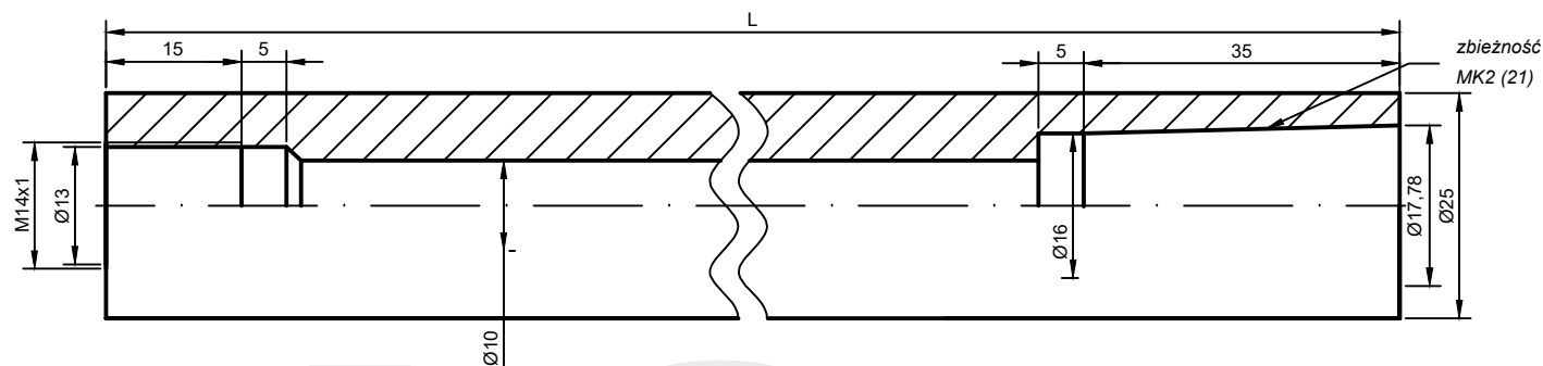
AW: S_21-25.L
