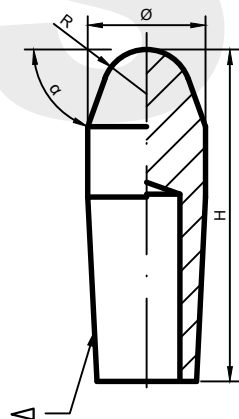
AW: Ek(R)-Ø.H- ▽
