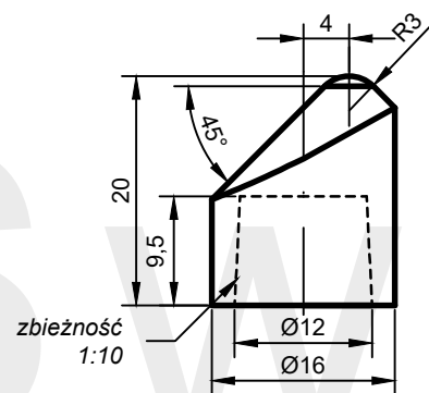
AW: N-D16(R3)*
