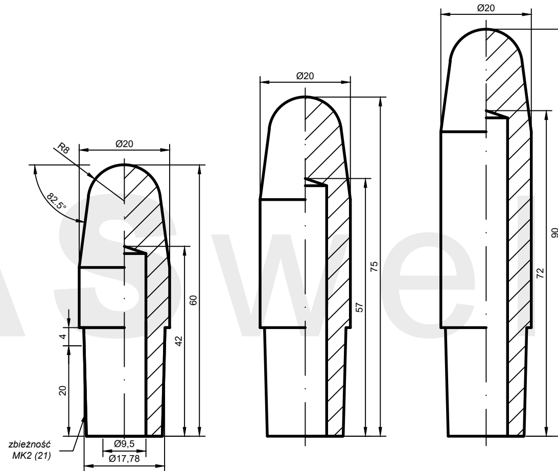
AW: E4(8)-20.60-21
