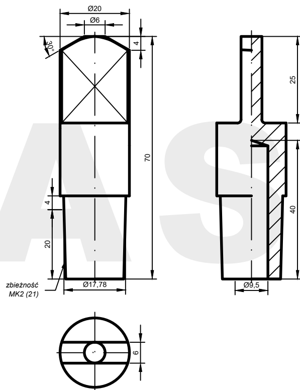
AW: B(6)-20(20x6).70-21*
