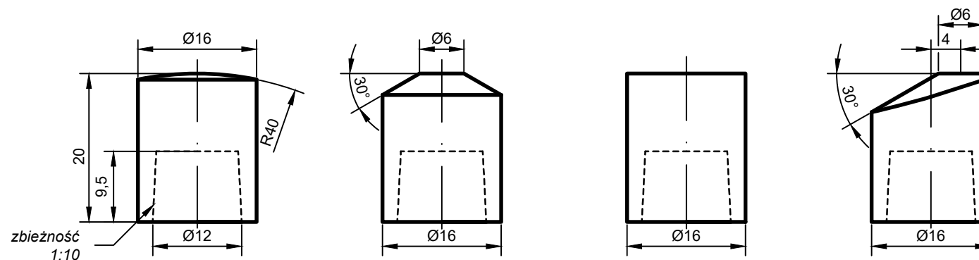
Typ: N-A16
