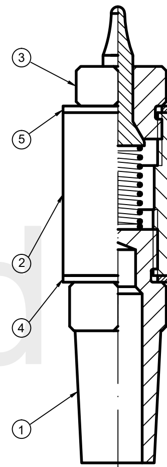
Elektroda z pinem do automatycznego podawania nakrętek
