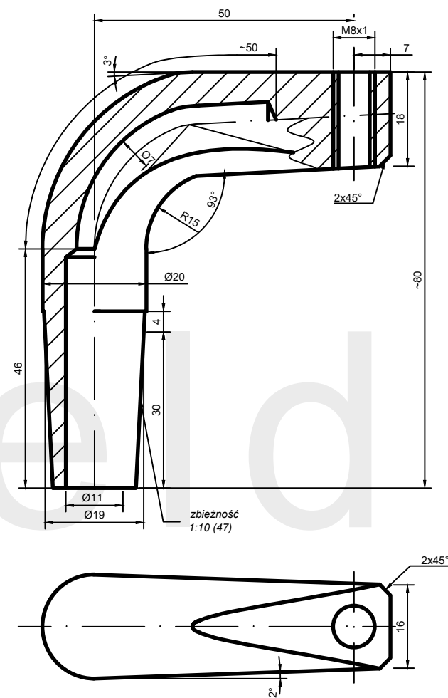
AW: GN8M1-20.80.50-47 *wykonanie na zamówienie
